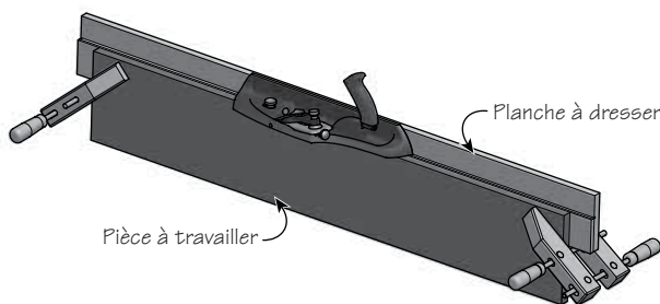
Figure 7 : Planche à dresser
