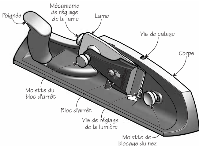
Figure 1 : Rabot pour planche à recaler Veritas
