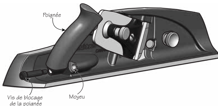
Figure 4 : Réglage de la poignée
