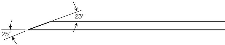
Figure 5 : Géométrie du tranchant de la lame
